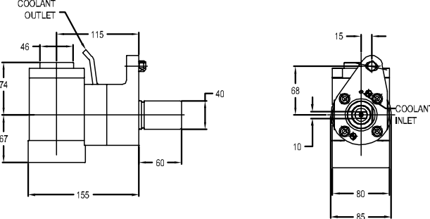
图纸：4 319.15680.000
