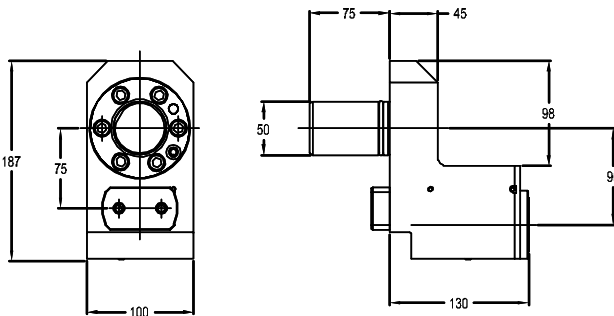
图纸：41 C5-L/RCE-MZ630-090130M
