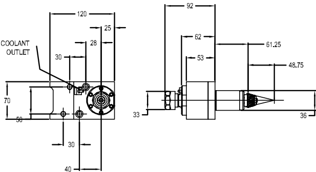
图纸：4 259.15620.000
