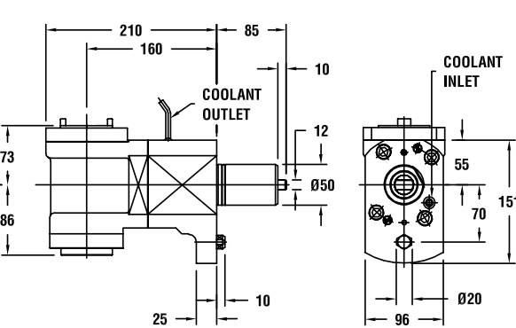
图纸：108 222.15654.000, 222.15658.000
