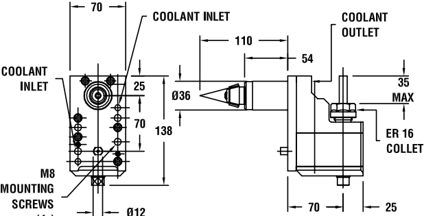
图纸：8 259.15613.000
