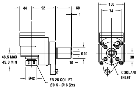
图纸：46
