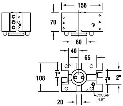
图纸：12 T00199
