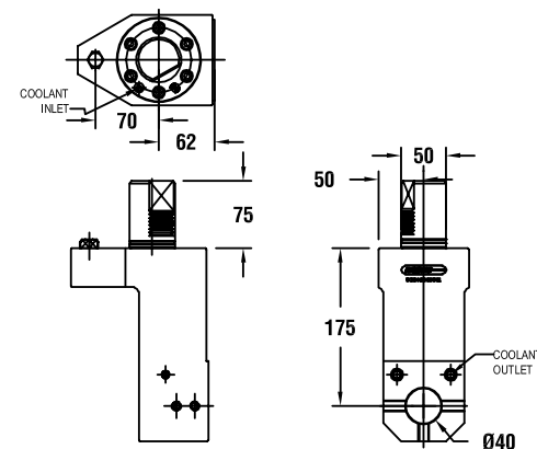
图纸：115 53308000501
