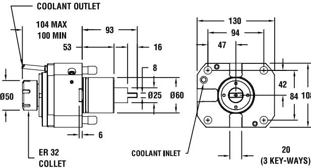
图纸：1 T32206
