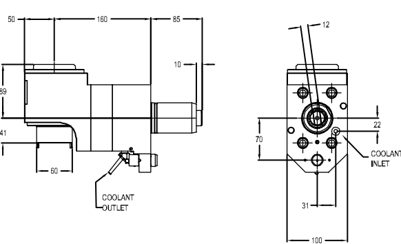
图纸：110 222.30010.000, 222.30020.000
