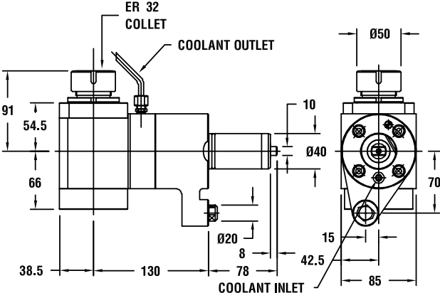
图纸：79 190.20010.000
