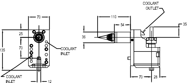
图纸：9 259.15614.000
