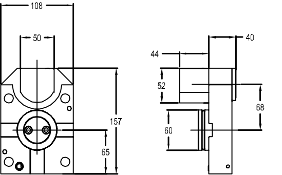
图纸：42 C4-L/RCE-NL2000-0680405A
