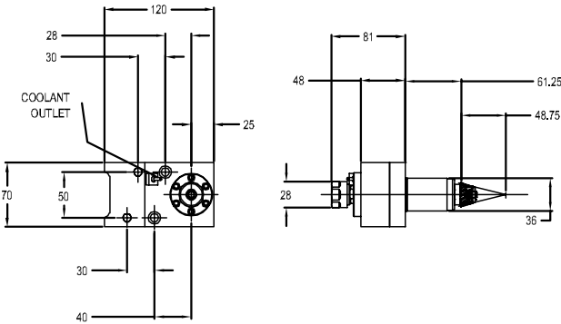
图纸：6 259.15624.000
