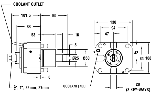
图纸：6 T32217
