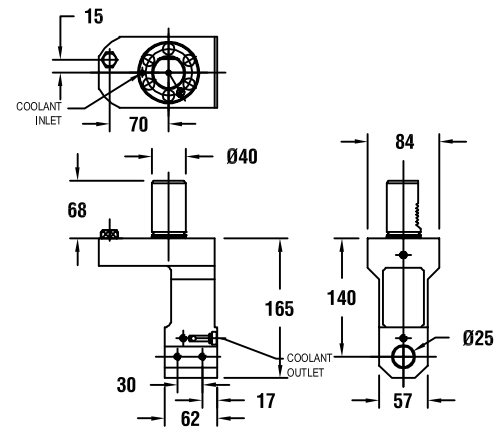
图纸：16 53478000400
