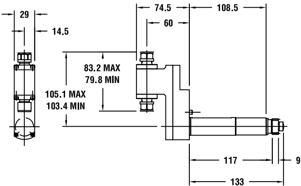
图纸：35 258.15986.000
