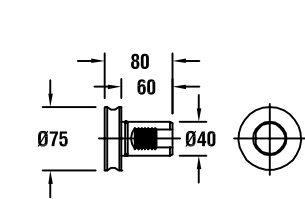
图纸：95 53518000600
