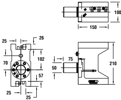
图纸：130 53838010800
