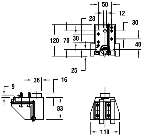
图纸：23 259.15909.000
