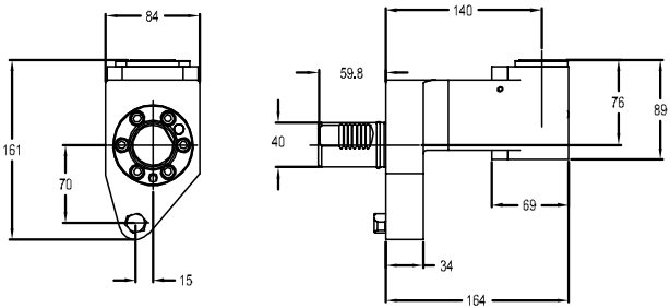
图纸：102 C4-L/RCI-SQT250-140076M
