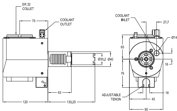
图纸：6 59-6353
