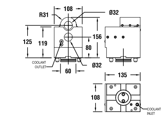
图纸：24 T10096
