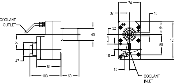
图纸：2 319.15679.000
