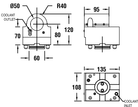
图纸：17 T10098
