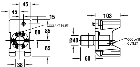
图纸：53 53518010100
