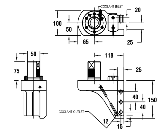
图纸：30 53488001001
