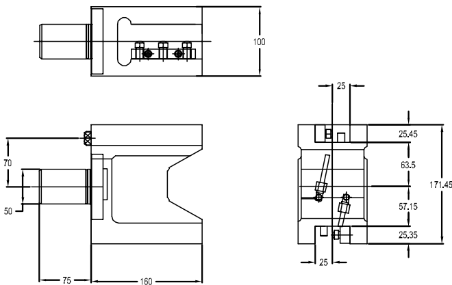
图纸：132 5333802010C1
