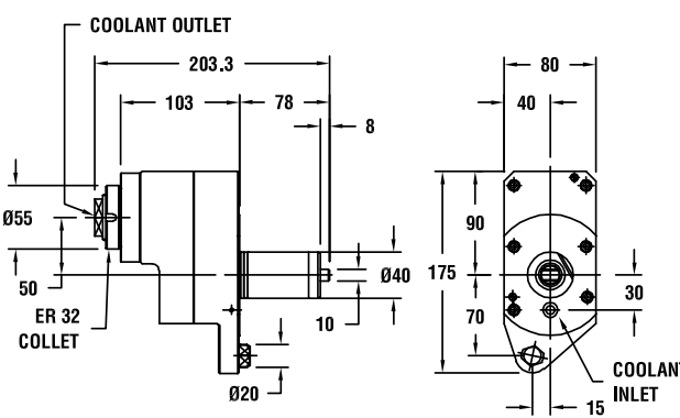
图纸：77 190.90010.000
