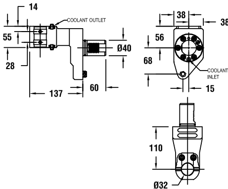
图纸：57 53518000201
