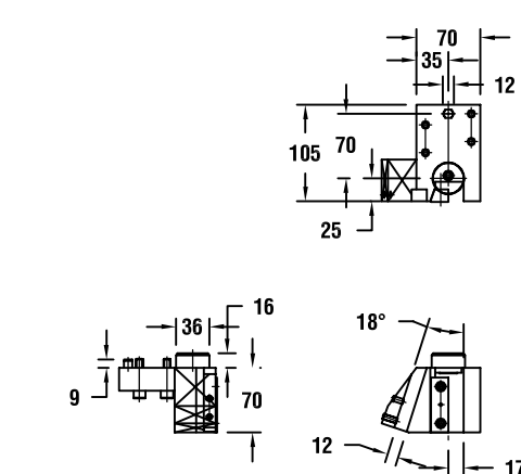
图纸：20 259.15444.000
