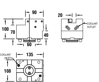
图纸：31 T03006
