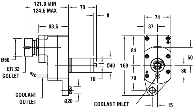
图纸：69 190.15685.000
