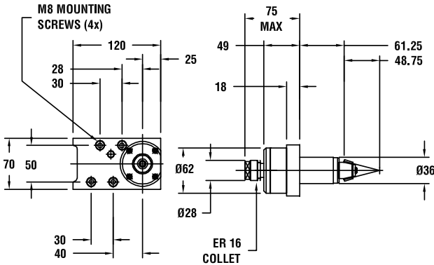
图纸：5 259.15622.000
