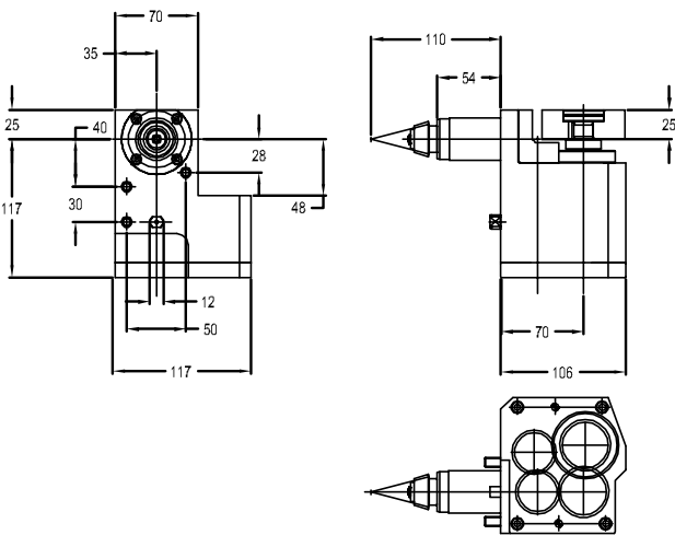
图纸：16 259.15789.000
