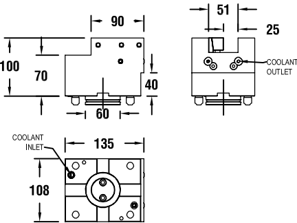
图纸：32 T03013
