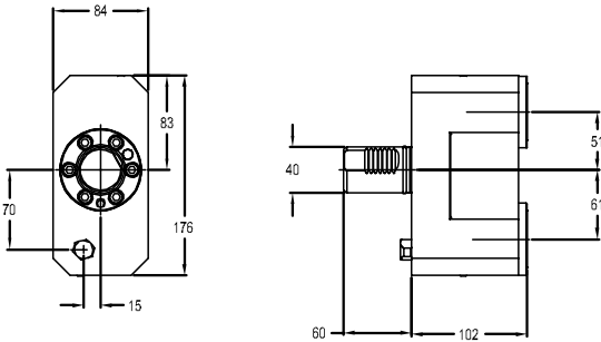
图纸：101 C5-L/RCE-SQT250-000102MDT
