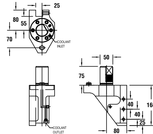
图纸：111 53308000101
