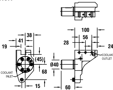
图纸：49 53518010100
