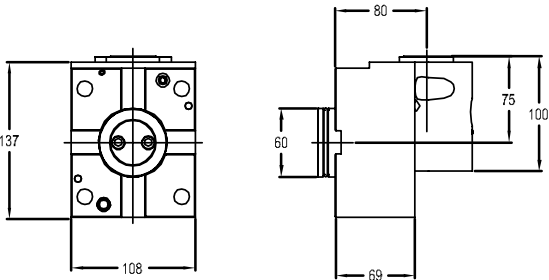
图纸：46 C4-L/RCI-NL2000-080075A
