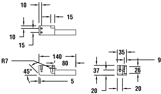
图纸：40 T17004
