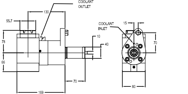
图纸：8 309.15088.000
