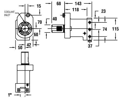
图纸：15 53478000900
