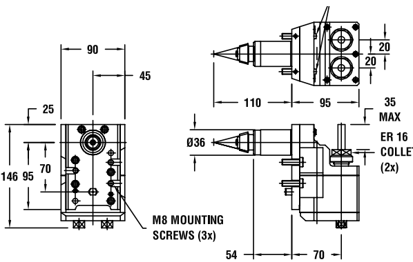
图纸：26 259.15907.000
