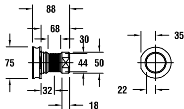
图纸 : 127 53818000701
