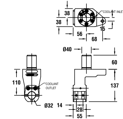
图纸：58 53538010200
