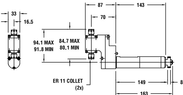
图纸：30 000.15172.000
