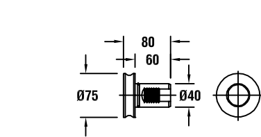
图纸：62 53518000600
