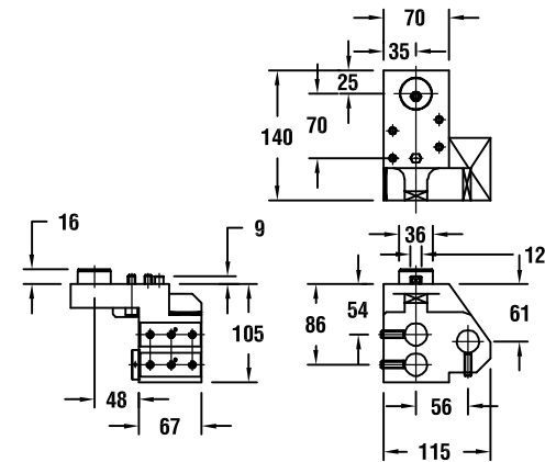
图纸：17 259.15443.000
