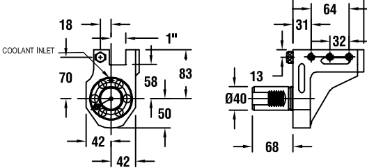
图纸：12 53478005100
