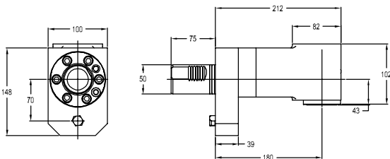
图纸：137 C5-L/RCE-SQT30-180043MSS
