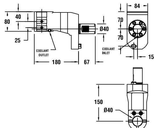
图纸：17 53478002100
