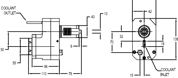
图纸：6 309.15089.000
