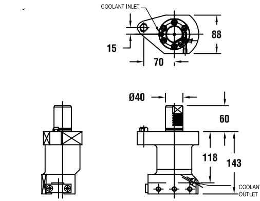
图纸：88 53618010300
