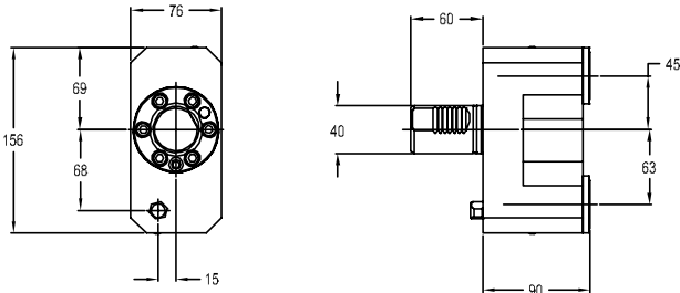
图纸：100 C4-L/RCE-SQT250-000099MDT
