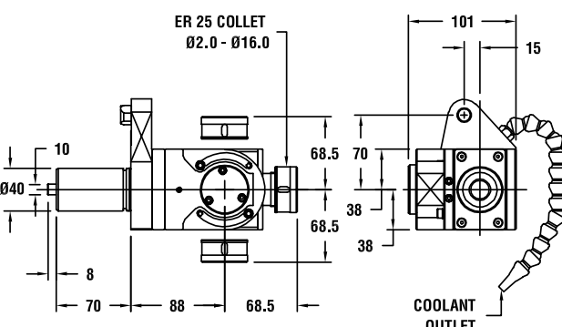
图纸：76 196.13989.000
