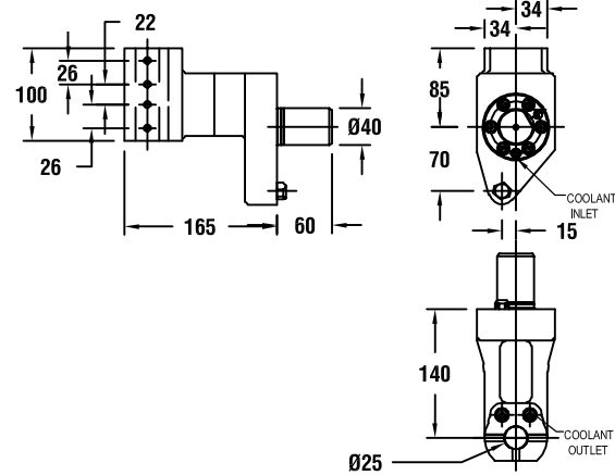
图纸：93 53638010400
