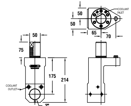
图纸：112 53308000201
