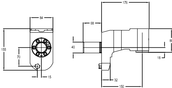
图纸：24 C4-L/RCI-MZ6200-150018M
