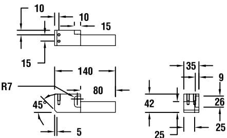
图纸：38 T17002
