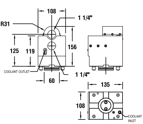
图纸：25 T10100
