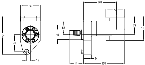
图纸：103 C5-L/RCI-SQT250-140079M
