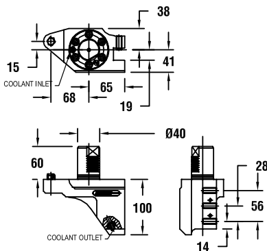
图纸：51 53518010700
