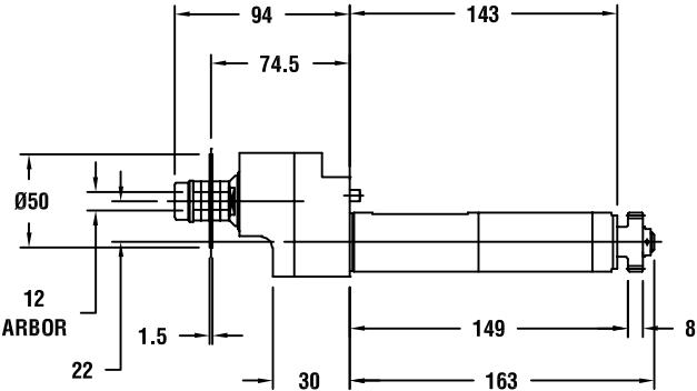
图纸：27 000.15700.000
