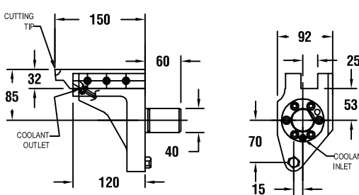
图纸：83 53618000600
