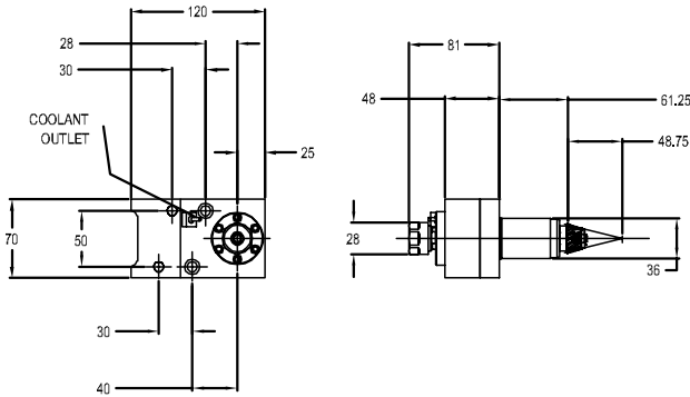
图纸：5 259.15622.000
