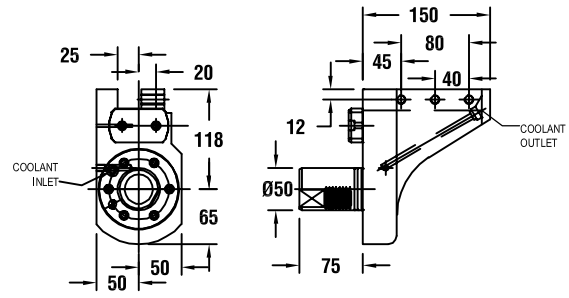
图纸：28 53488001101
