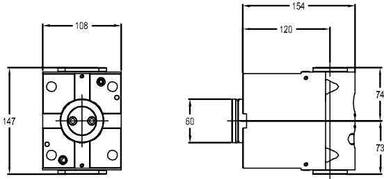
图纸：50 C4-L/RCE-NL2000-125075ADT
