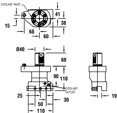
图纸：55 53518010300
