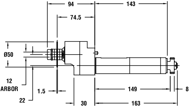
图纸：28 000.15964.000
