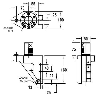
图纸：116 53308000601
