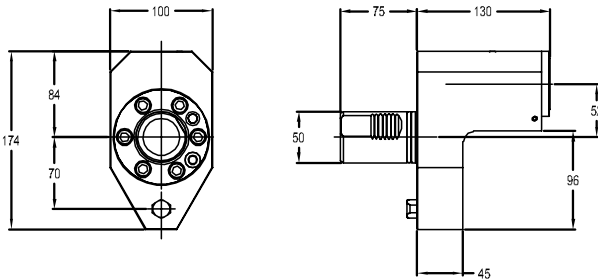
图纸：133 C5-L/RCE-SQT30-052130M
