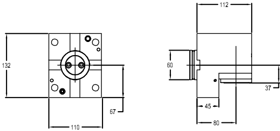
图纸：48 C5-L/RCI-NL3000-080037A
