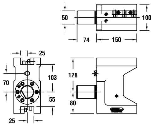
图纸 : 128 53838000801
