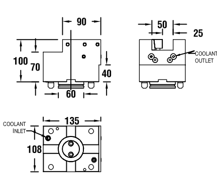
图纸：30 T03005
