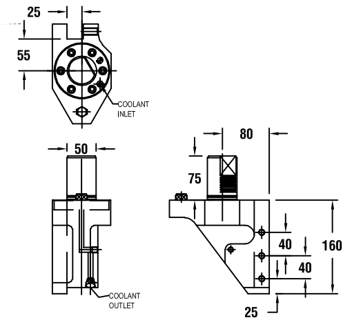
图纸 : 117 53308010100
