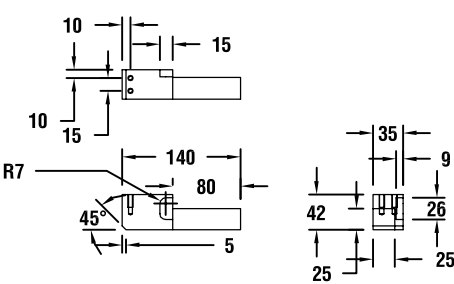
图纸：39 T17003
