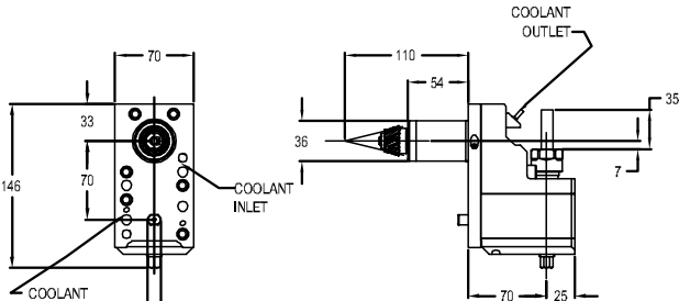
图纸：10 259.15615.000
