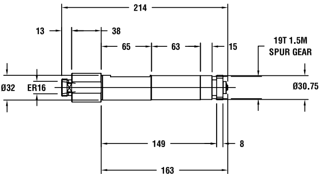
图纸：29 000.15182.000
