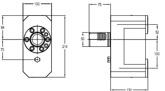
图纸：135 C5-L/RCE-SQT30-000130MDT
