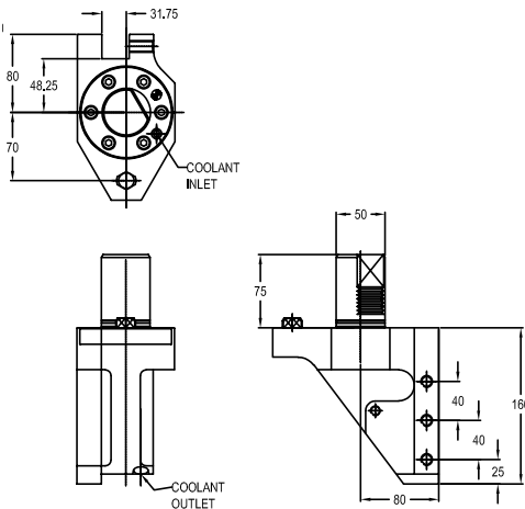
图纸 : 127 53818000701
