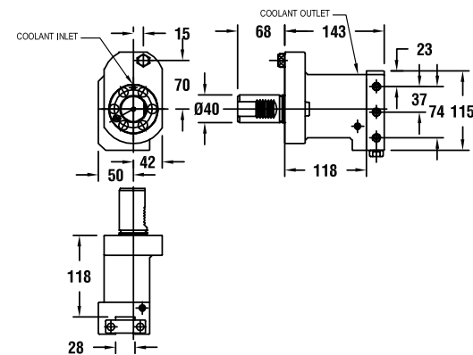
图纸：16 53478000400
