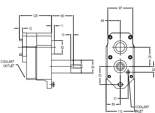
图纸：107 222.15700.000, 222.15710.000
