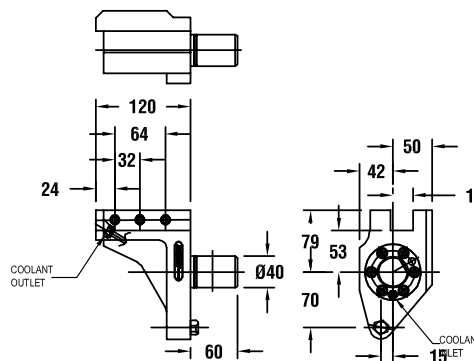
图纸：84 53618010600
