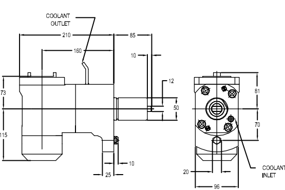
图纸：109 222.15720.000, 222.15730.000
