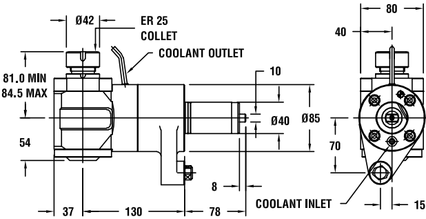
图纸：71 190.15665.000
