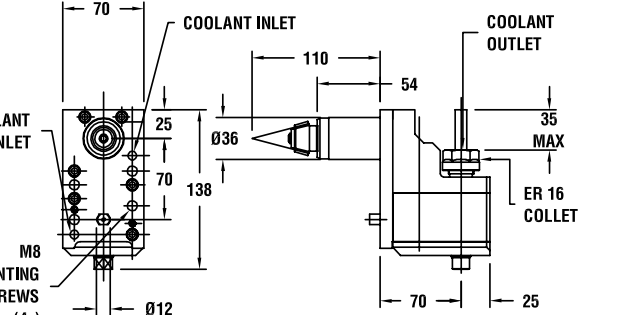
图纸：12 259.15708.000
