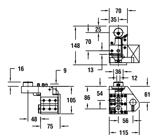
图纸：19 259.15612.000
