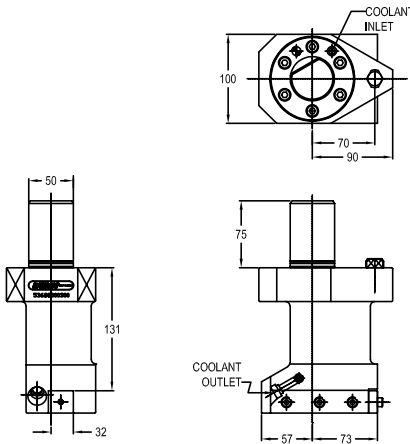
图纸 : 123 53688000300
