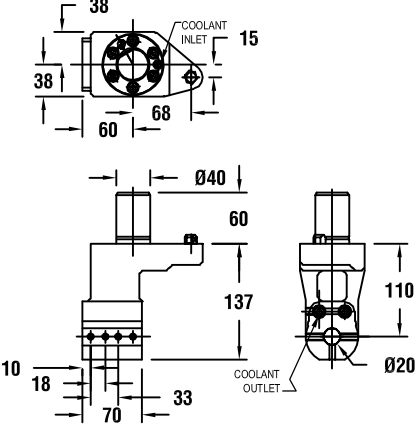
图纸：60 53518010200
