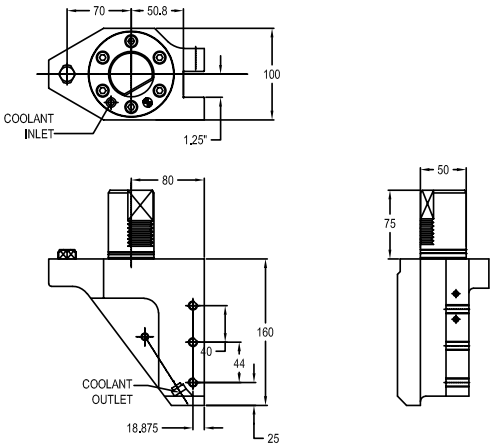
图纸 : 124 53688010100
