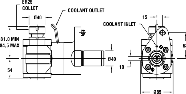
图纸：3 319.15660.000
