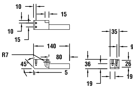
图纸：41 T17005
