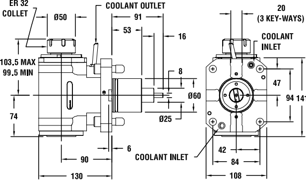
图纸：3 T32207
