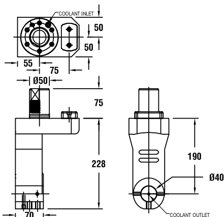
图纸：39 53488001801
