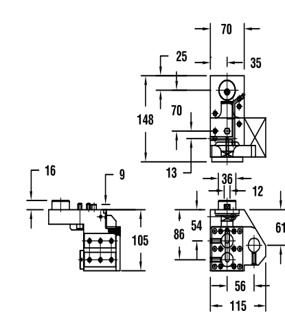
图纸：18 259.74010.000
