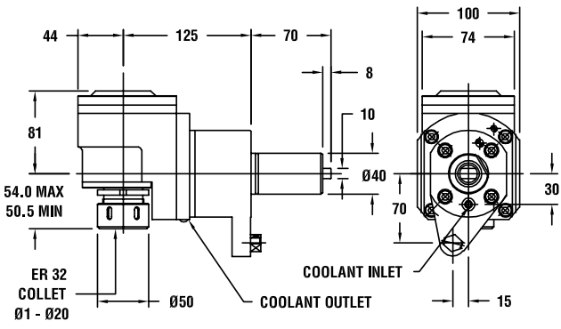
图纸：74 190.14718.000
