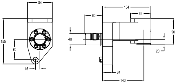
图纸：104 C4-L/RCI-SQT250-140020MSS
