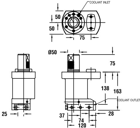
图纸：33 53488006401
