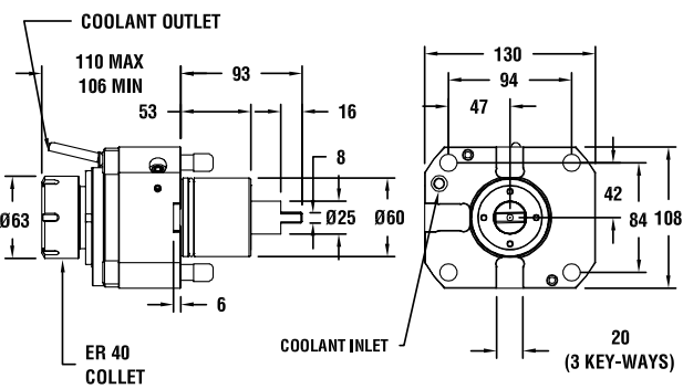
图纸：4 T32214
