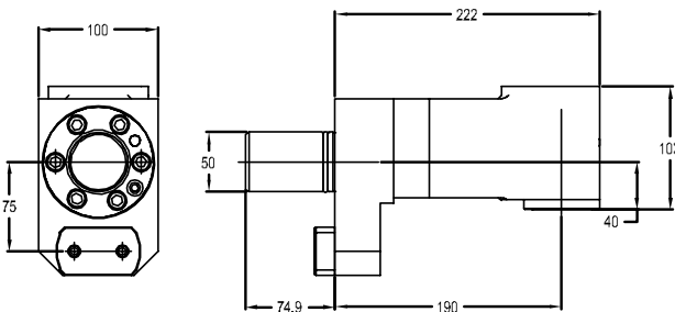
图纸：42 C5-L/RCI-MZ630-190040M
