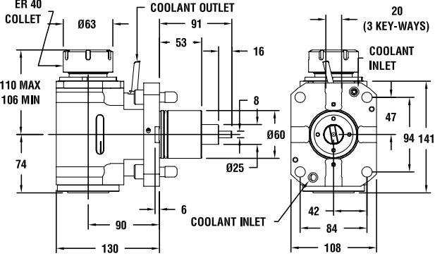
图纸：4 T32214
