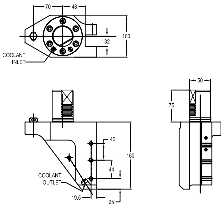
图纸 : 121 53688000100
