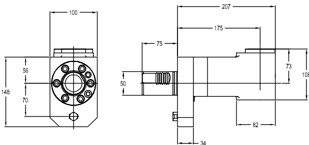
图纸：136 C5-L/RCI-SQT30-175073M
