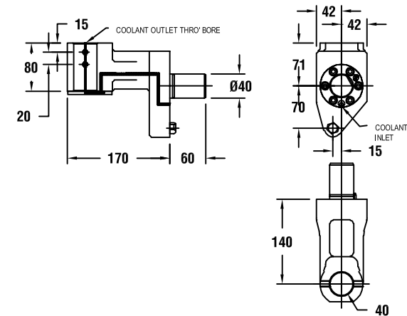
图纸：94 53208005200
