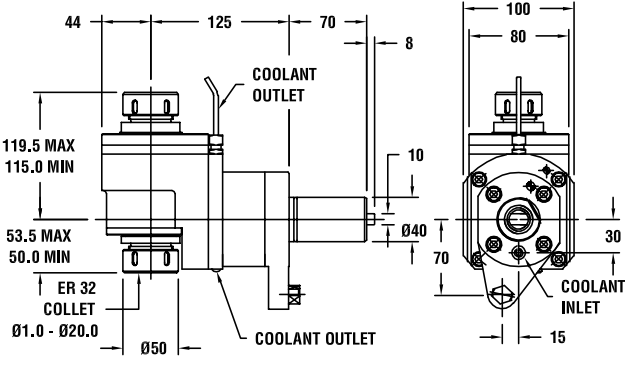
图纸：75 190.14823.000
