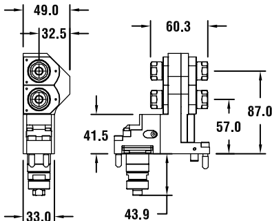
图纸：1 GSE2007
