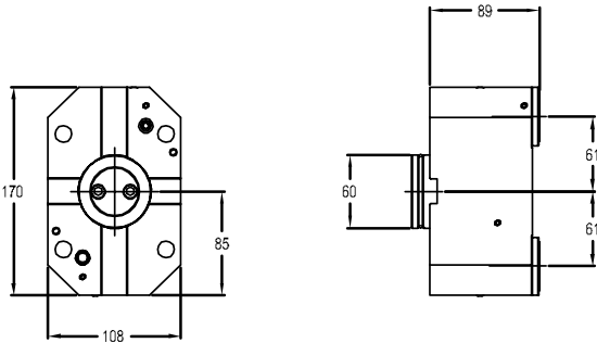
图纸：49 C4-L/RCE-NL2000-061089ADT
