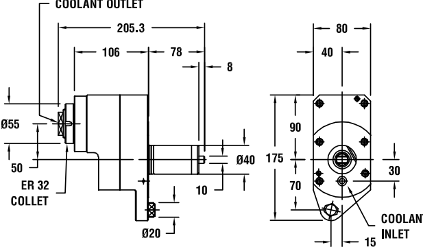
图纸：78 190.10020.000
