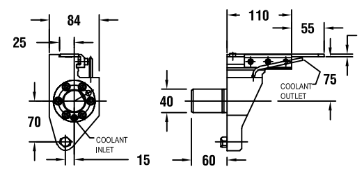
图纸：89 53618000400
