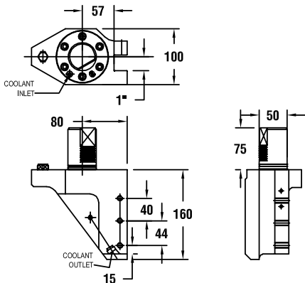
图纸 : 120 53308010600
