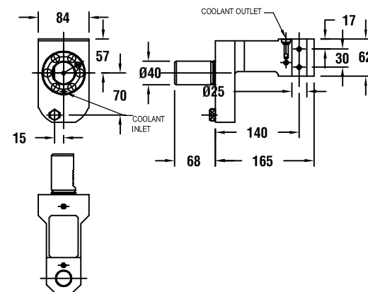
图纸：18 53478005400
