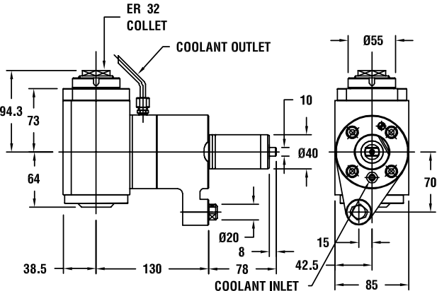
图纸：80 190.90020.000
