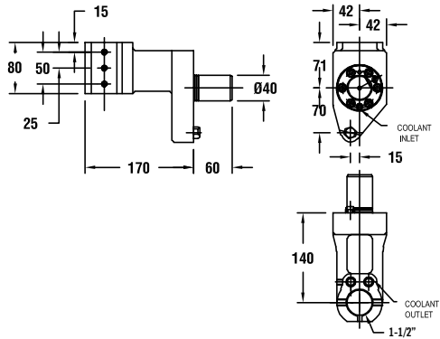
图纸：91 53208015100
