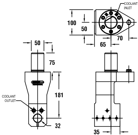
图纸：129 5383800901
