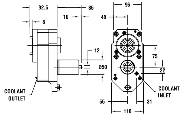
图纸：106 222.15653.000, 222.15656.000
