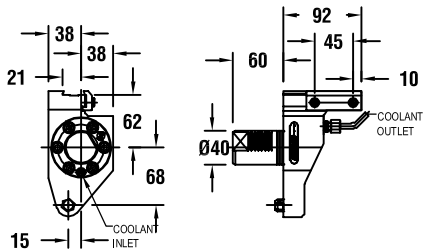
图纸：56 53518000401
