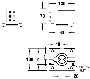
图纸：14 T00202
