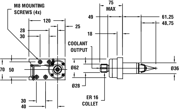
图纸：7 259.15707.000
