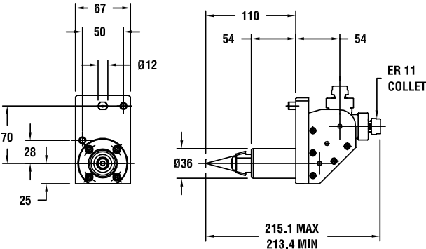
图纸：13 259.15441.000
