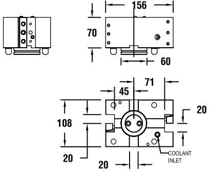
图纸：9 T00185
